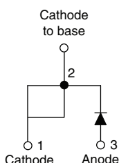
TO-220AC
