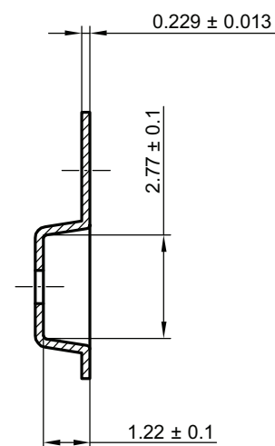
A-A Section
