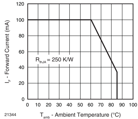
図 2 - 順方向電流限界 対 周囲温度
