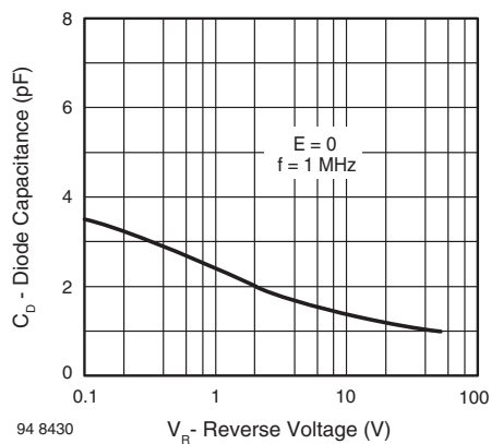
図 4 - 端子間容量 VS. 逆電圧
