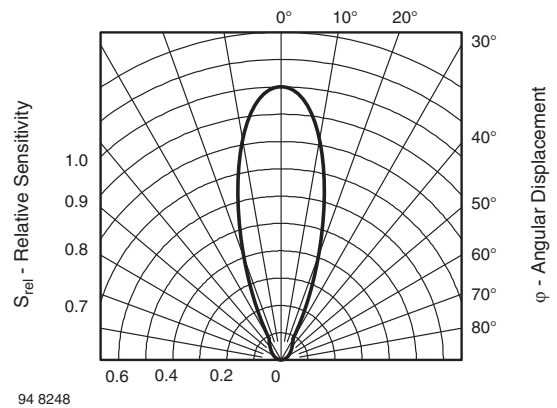
図 6 - 相対放射強度 対 角変位
