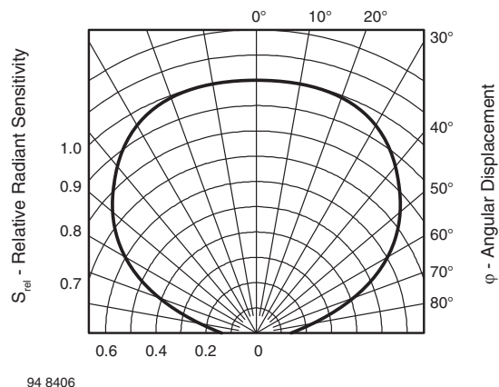
図 7 - 相対放射感度 VS. 角変位
