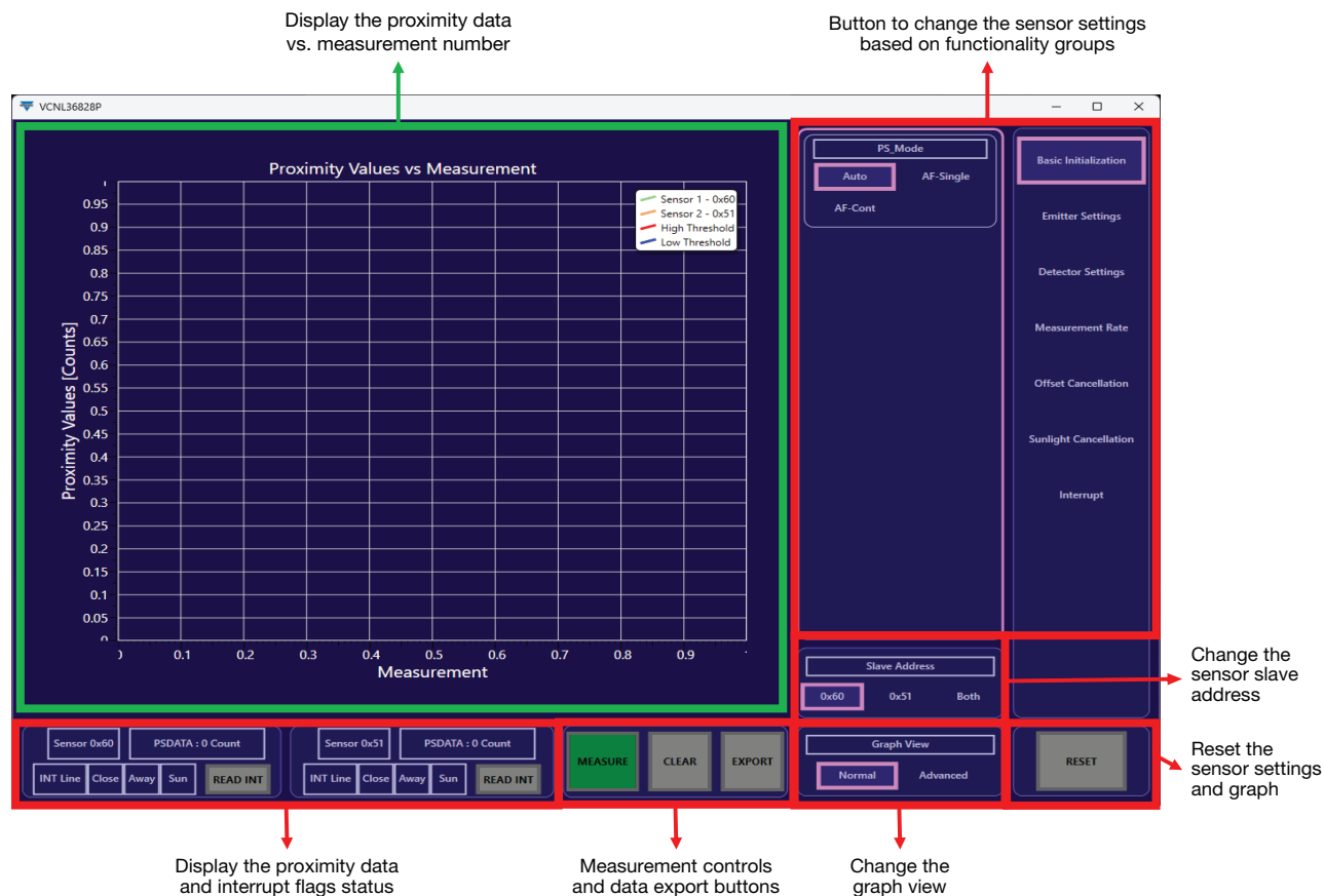
Fig. 2 - Demosoftware GUI
