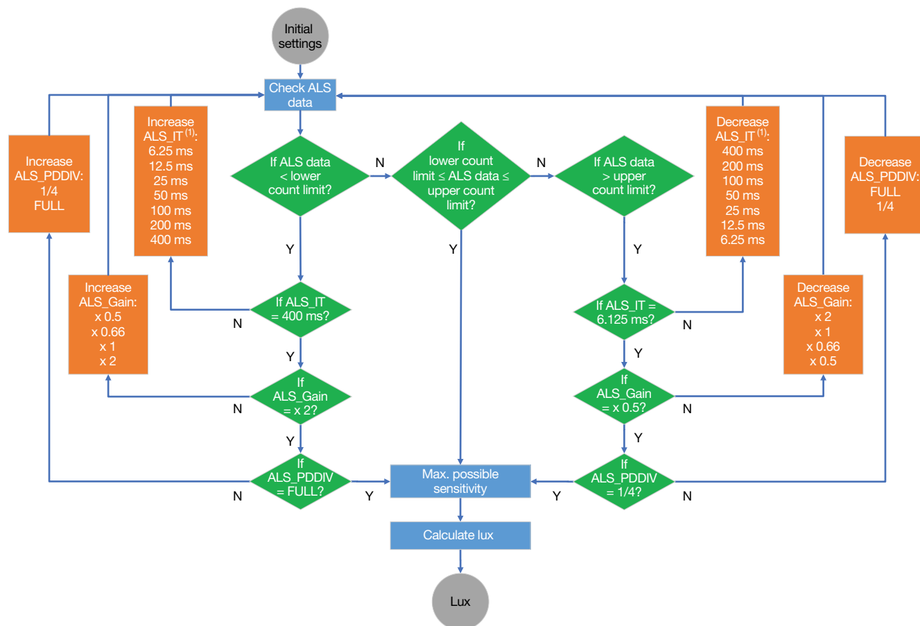
Fig. 6 - VEML4031X00 AGC
