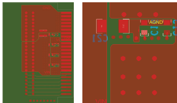
Fig. 21 - Bottom Layer
