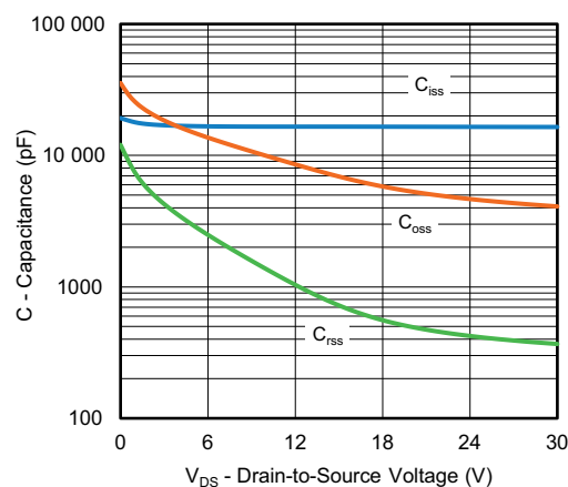
Fig. 4 - Capacitance
